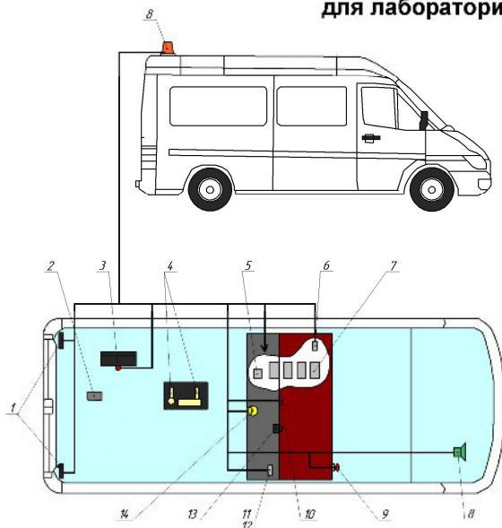
Схема расположения элементов электробезопасности для лаборатории ЛВИ НВТ
