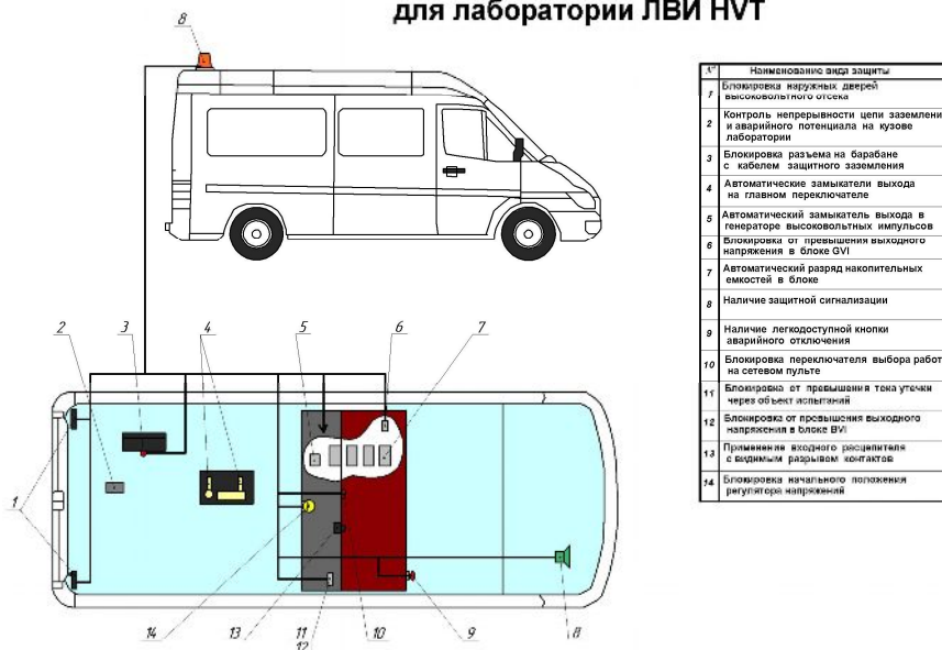
Схема расположения элементов электробезопасности для лаборатории ЛВИ НУТ
