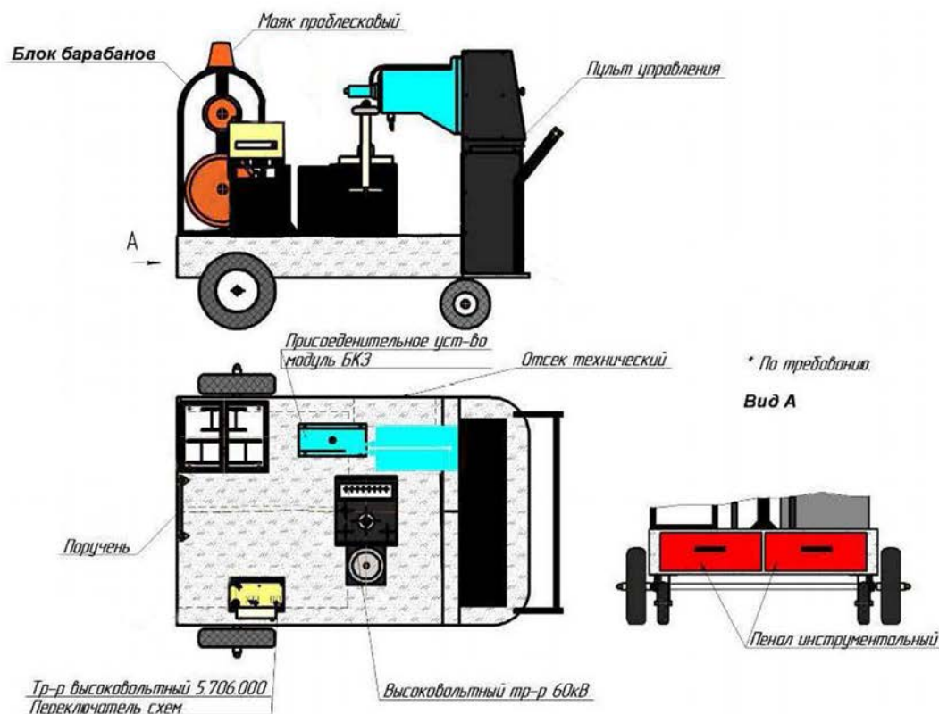
Рис.1 Планировка микролаборатории МИЛЯ-3
